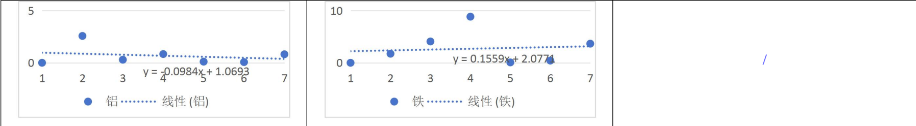
图10.2-2 地下水GW2点位污染物浓度监测值变化及趋势预测图
