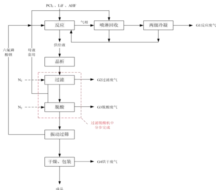
图 4.1-1 生产工艺流程简图
